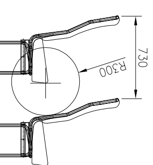
DETALHE ESPAÇAMENTO POLTRONAS
